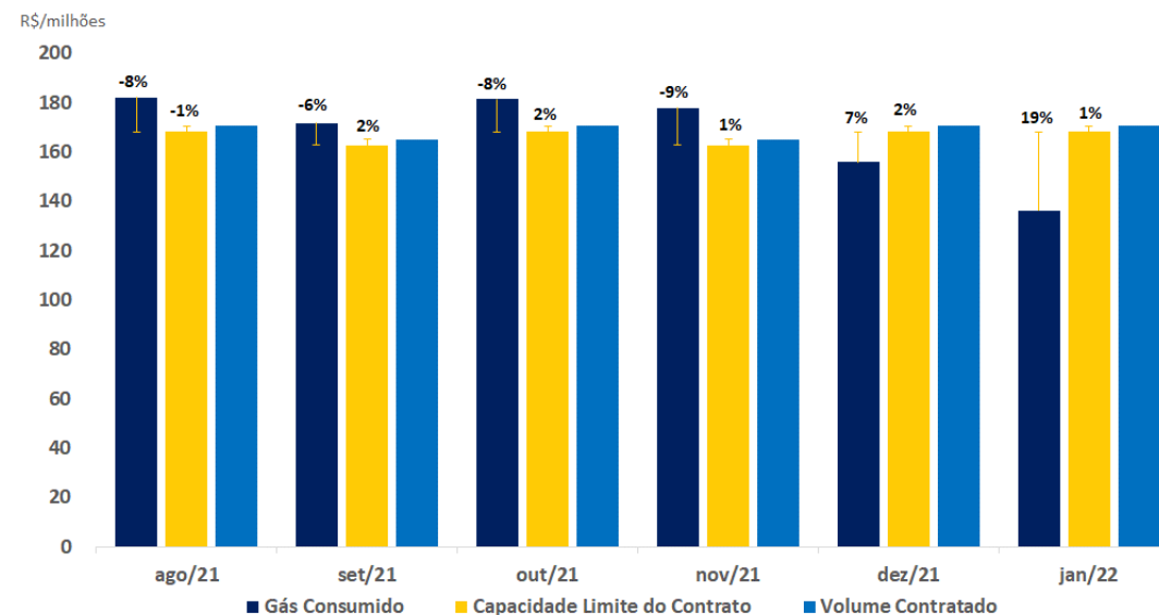
Gráfico 14 – Consumo x Capacidade x Contrato
