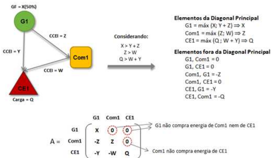
Figura 5: Exemplo de Montagem da Matriz de Comercialização de Energia Incentivada
