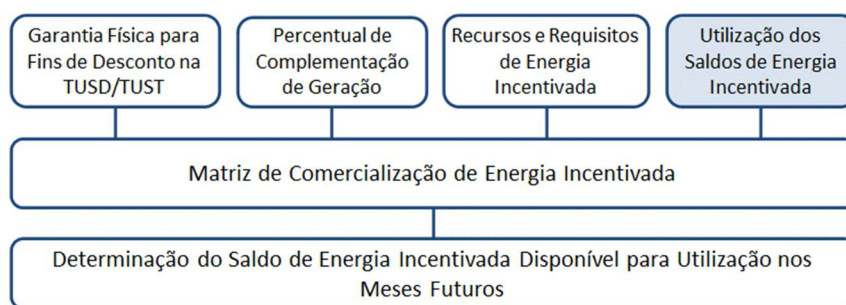
Figura 10: Esquema Geral do Módulo “Cálculo do de Descontos Aplicado à TUSD/TUST”
