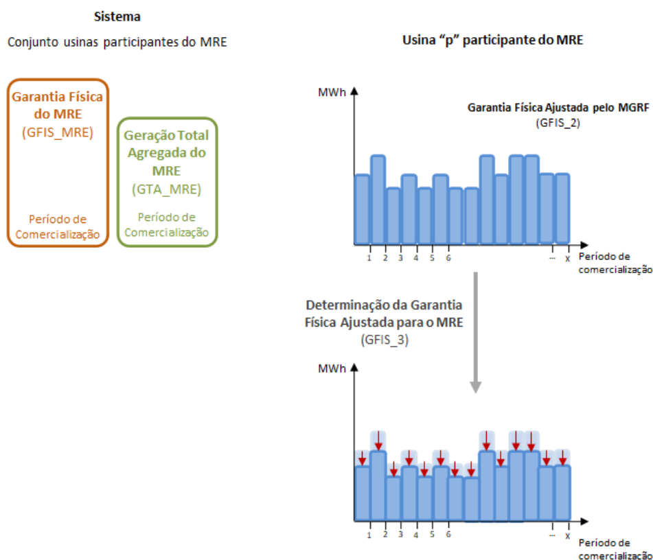
Figura 8: Representação gráfica do processo de Determinação da Garantia Física Modulada Ajustada para o MRE
