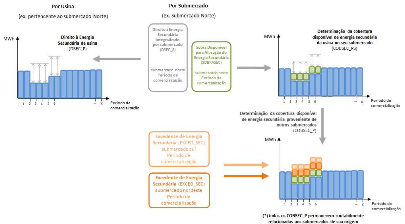
Figura 21: Representação gráfica do processo de determinação da Cobertura Disponível de Energia Secundária da usina
