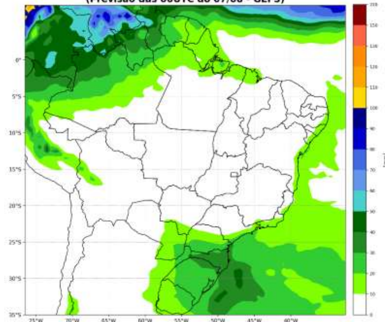
Precipitação acumulada (mm) entre os dias: 16/08 e 22/08 (semana 4) (Previsão das 00UTC do 07/08 - GEFS)
