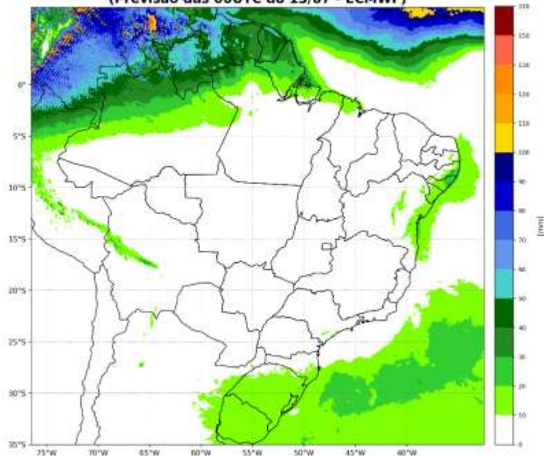
Precipitação acumulada (mm) entre os dias: 19/07 e 25/07 (semana 4) (Previsão das 00UTC do 13/07 - ECMWF)
