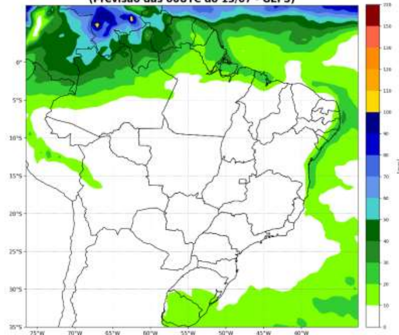
Precipitação acumulada (mm) entre os dias: 19/07 e 25/07 (semana 4) (Previsão das 00UTC do 13/07 - GEFS)
