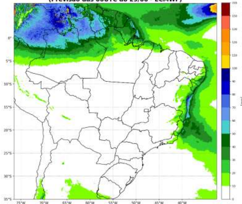
Precipitação acumulada (mm) entre os dias: 05/07 e 11/07 (semana 2) (Previsão das 00UTC do 29/06 - ECMWF)
