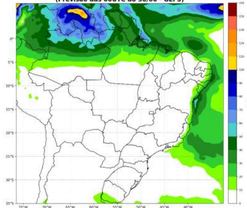
Precipitação acumulada (mm) entre os dias: 05/07 e 11/07 (semana 2) (Previsão das 00UTC do 30/06 - GEFS)
