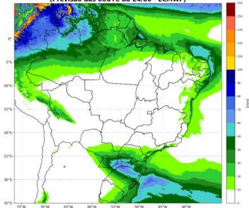
Precipitação acumulada (mm) entre os dias: 28/06 e 04/07 (semana 1) (Previsão das 00UTC do 24/06 - ECMWF)
