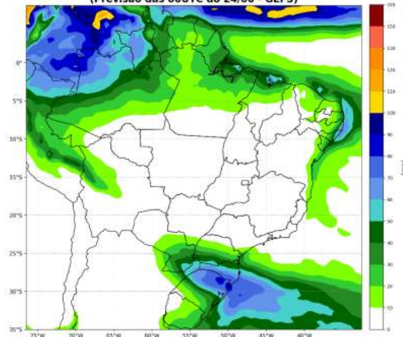
Precipitação acumulada (mm) entre os dias: 28/06 e 04/07 (semana 1) (Previsão das 00UTC do 24/06 - GEFS)
