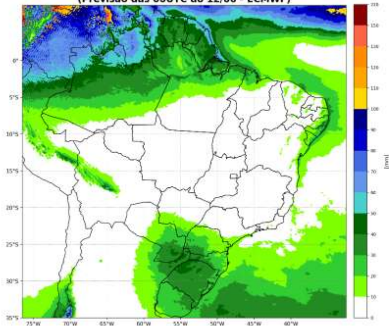
Precipitação acumulada (mm) entre os dias: 21/06 e 27/06 (semana 4) (Previsão das 00UTC do 12/06 - ECMWF)
