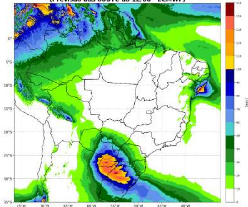
Precipitação acumulada (mm) entre os dias: 14/06 e 20/06 (semana 3) (Previsão das 00UTC do 12/06 - ECMWF)
