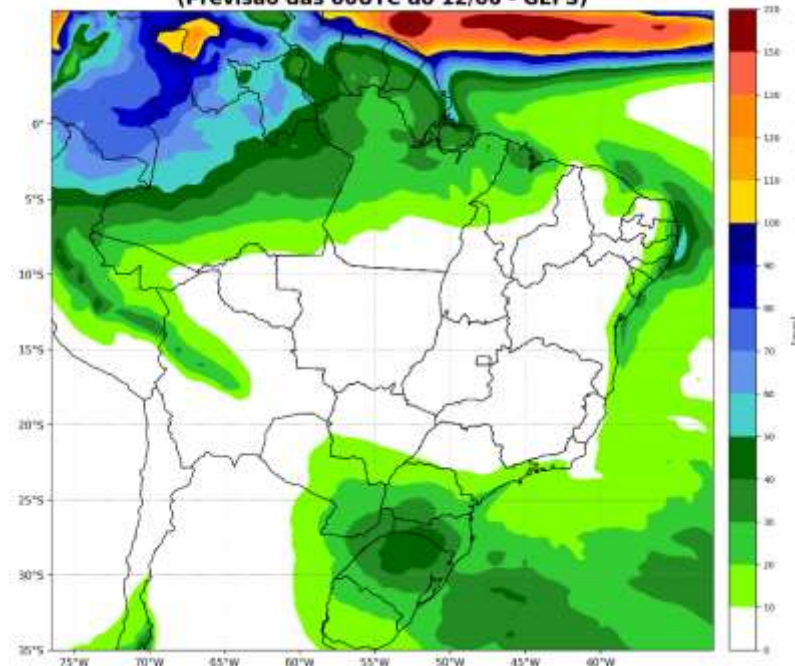
Precipitação acumulada (mm) entre os dias: 21/06 e 27/06 (semana 4) (Previsão das 00UTC do 12/06 - GEFS)
