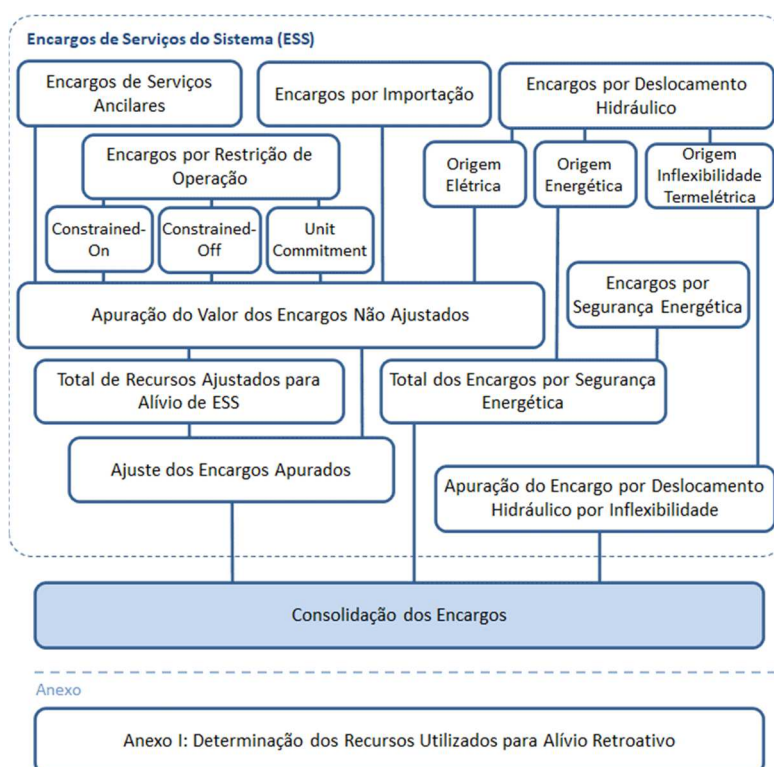
Figura 21 - Esquema Geral do Módulo de Regras: "Encargos"
