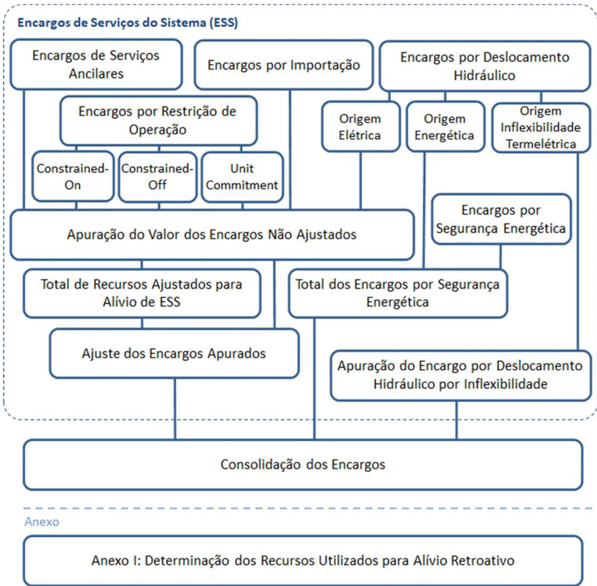
Figura 1: Esquema Geral do Módulo de Regras: “Encargos”
