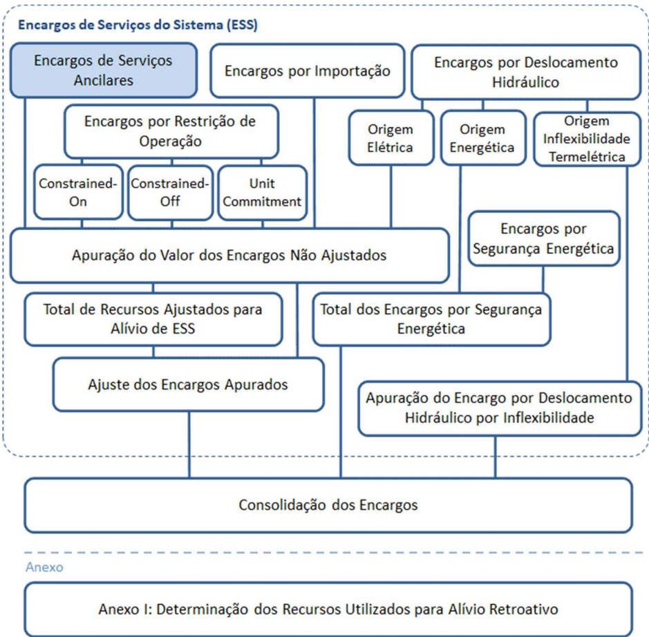
Figura 11: Esquema Geral do Módulo de Regras: “Encargos”
