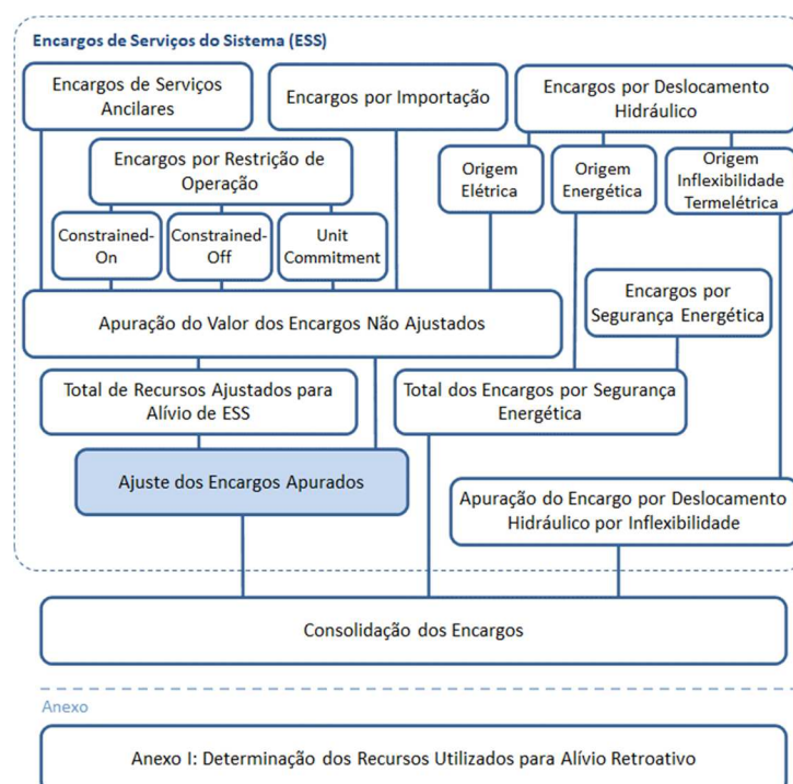
Figura 18: Esquema Geral do Módulo de Regras: "Encargos"
