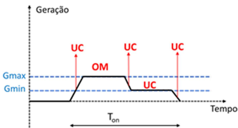
Figura 3 – Representação das Restrições Operativas por Unit Commitment
