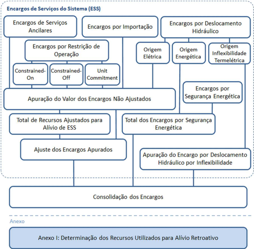
Figura 22: Esquema Geral do Módulo de Regras: “Encargos”
