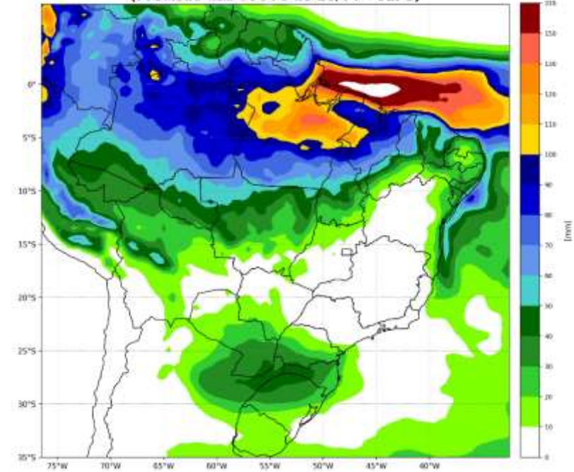
Precipitação acumulada (mm) entre os dias: 20/04 e 26/04 (semana 4) (Previsão das 00UTC do 18/04 - GEFS)
