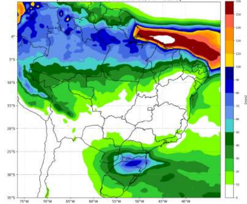
Precipitação acumulada (mm) entre os dias: 27/04 e 03/05 (semana 1) (Previsão das 00UTC do 18/04 - GEFS)
