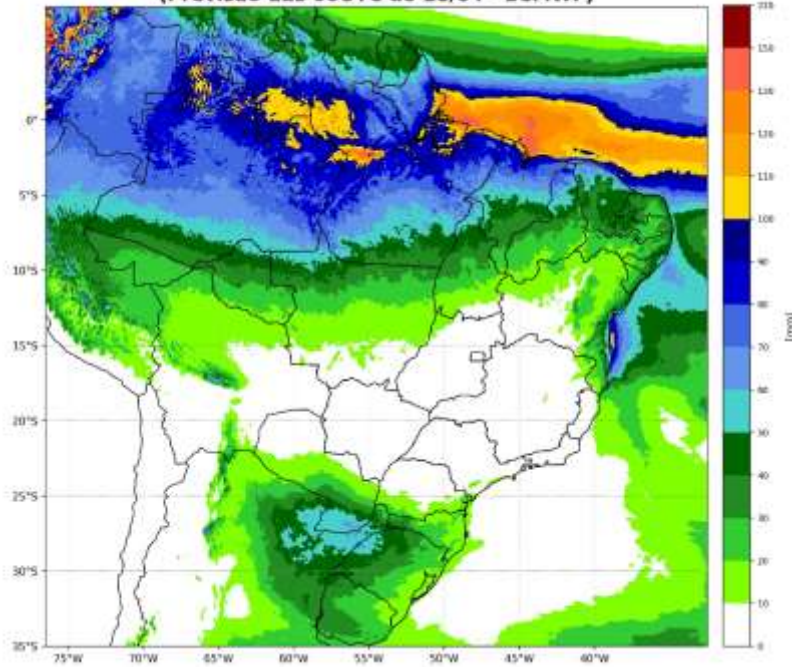
Precipitação acumulada (mm) entre os dias: 20/04 e 26/04 (semana 4) (Previsão das 00UTC do 18/04 - ECMWF)
