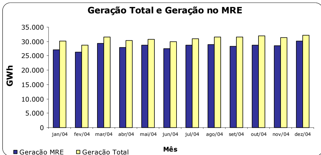
Gráfico 12 – Geração Total do Sistema e Geração no MRE
